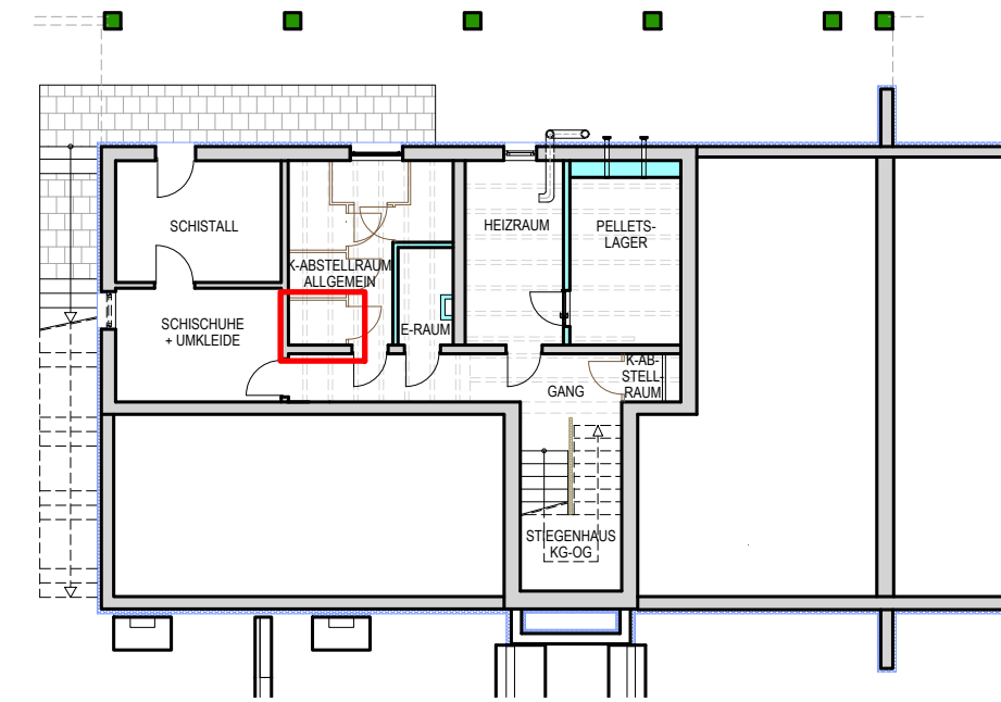
GRUNDRISS KELLERGESCHOSS M1:200
