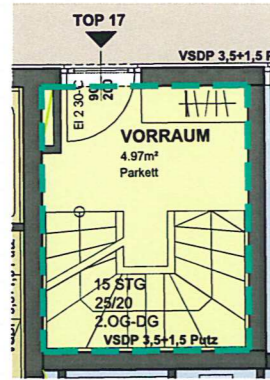
2. OBERGESCHOSS / TOP 17 / M=1:100
