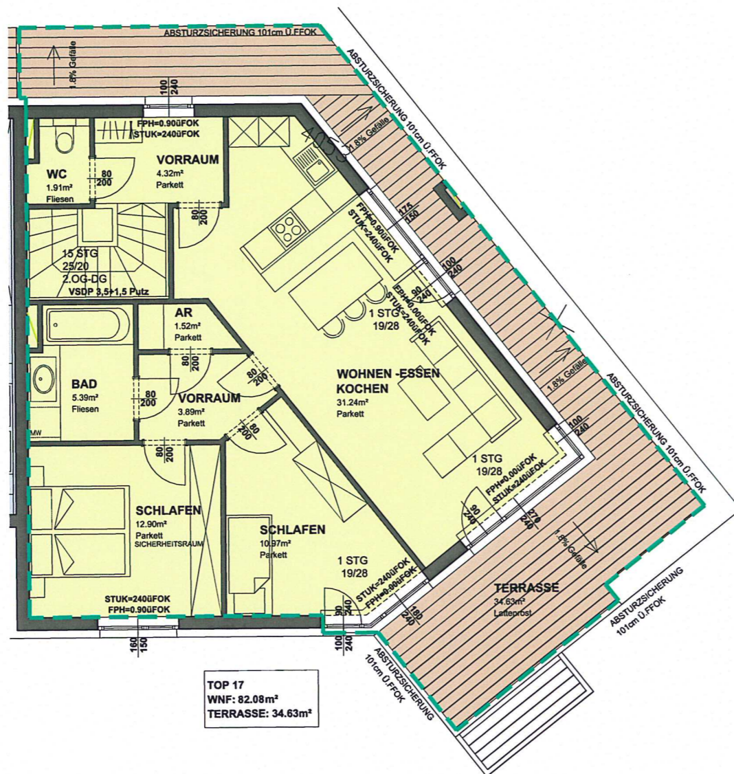
DACHGESCHOSS / TOP 17 / M=1:100
