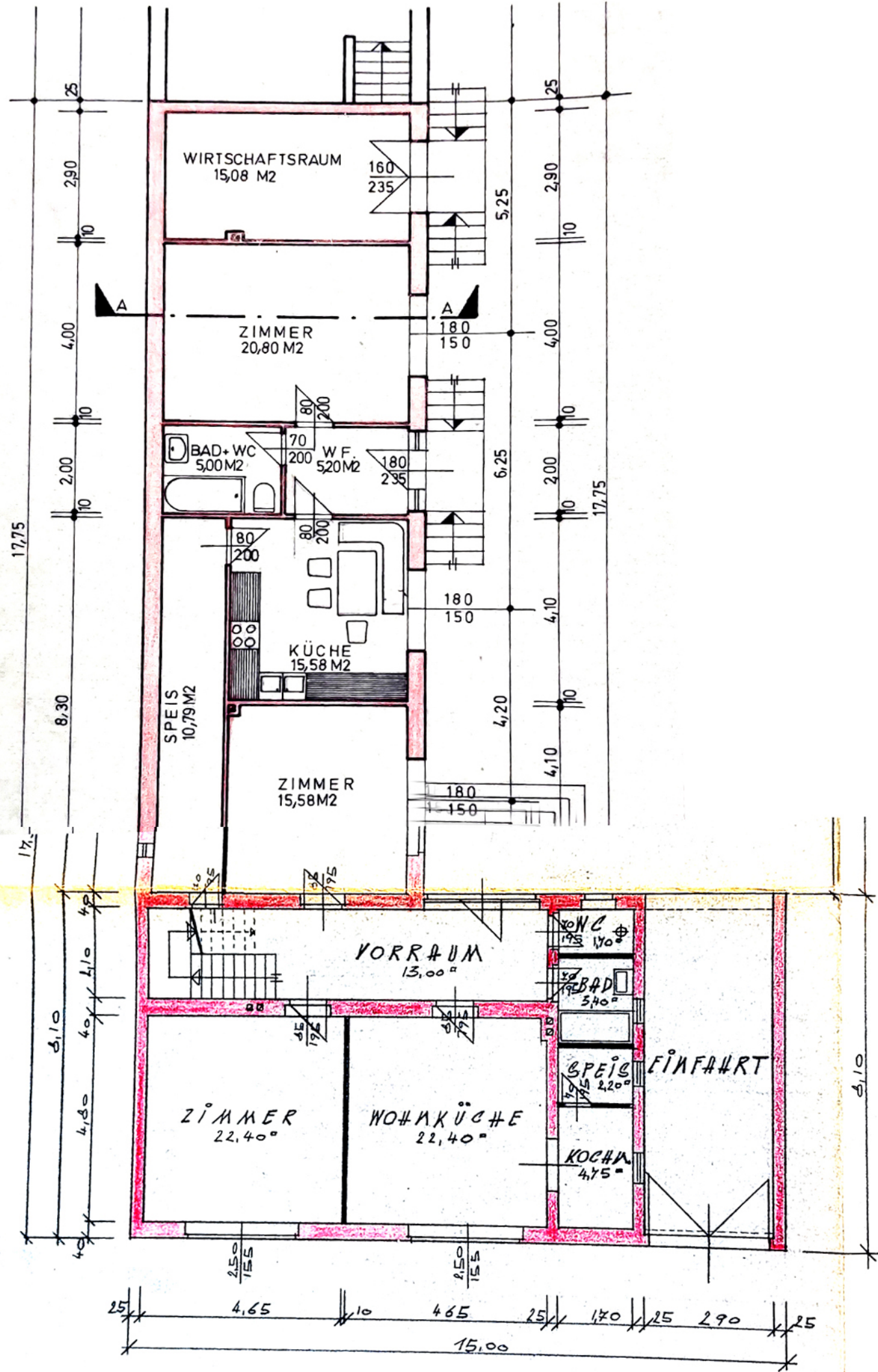
ERDGESCHOSS 1:100
