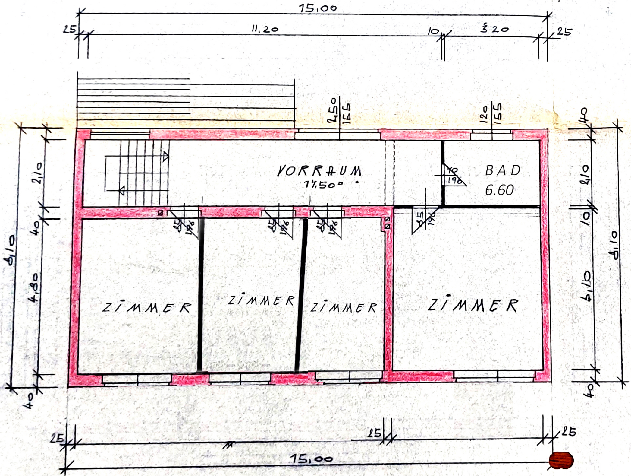
OBERGESCHOSS 1:100
