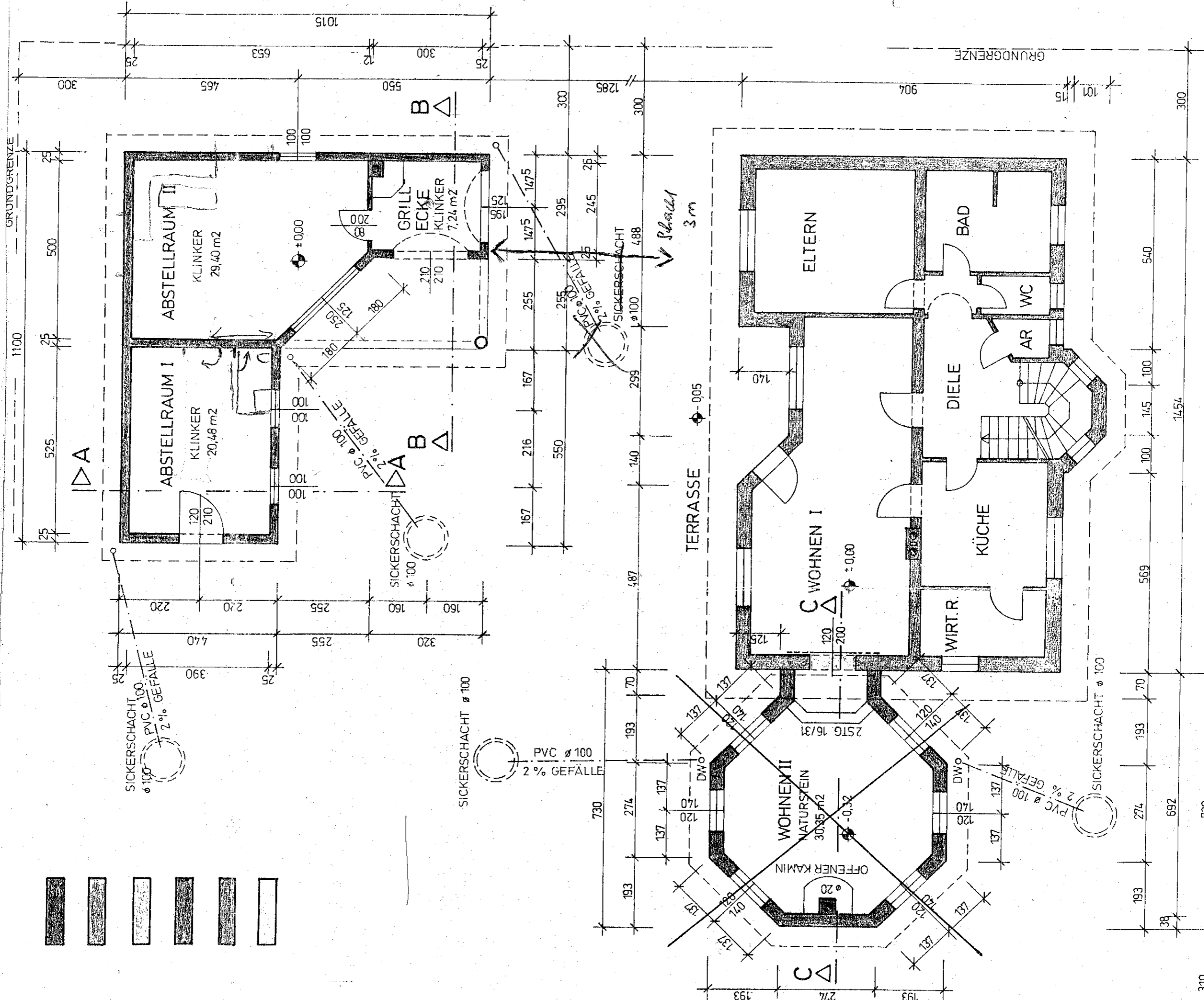
GRUNDRISS ERDGESCHOSS
